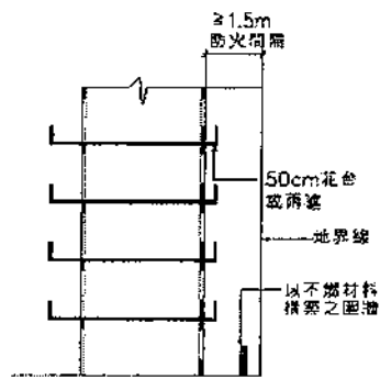
花台或雨蓬可突出防火間隔50cm，防火間隔範圍內得設置以不燃材料構築之圍牆。 第110條 圖110-(4)
